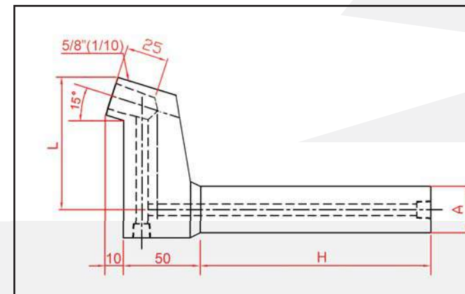
標準L型通水銅(L-holder)-15° Head
