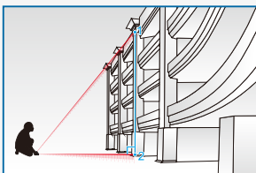
畢氏定理
