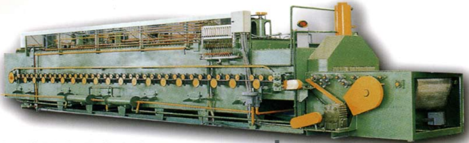
連續滲碳淬火爐
