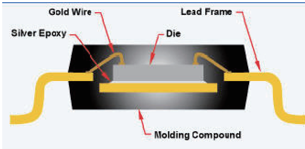
MSOP, Mini Small Outline Package
