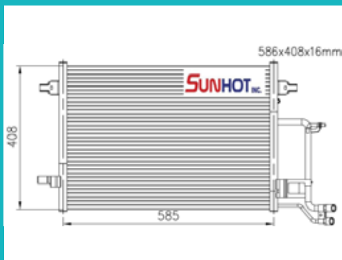
Audi A4 - CAD003 - Condenser
