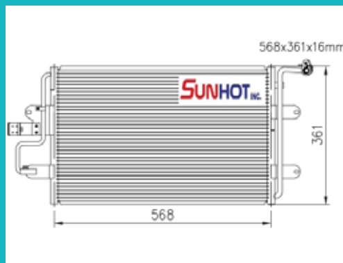
Audi A3 - CAD007 - Condenser
