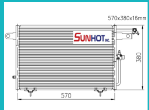
Audi A6 - CAD008 - Condenser
